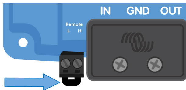
Connecteur d'allumage/arrêt à distance avec boucle de fil
