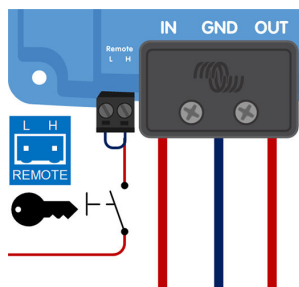
Diagramme de connexion pour ignorer la détection de moteur à l'arrêt
